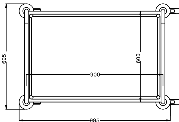
Boven aanzicht
